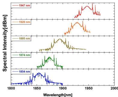
2 μm帯高出力Tm添加超短パルスファイバーレーザー
