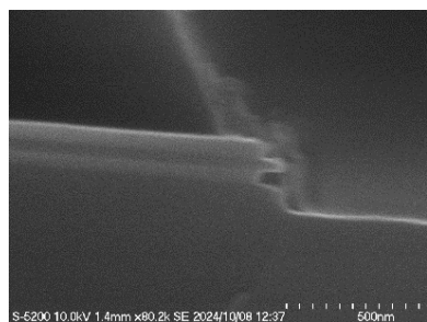
SiGe/Si/SiGe積層構造におけるSiGe選択エッチング
