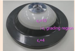
ガス絶縁開閉装置(GIS) 245kV-GIS用FGMスペーサ
