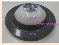
ガス絶縁開閉装置(GIS) 245kV-GIS用FGMスペーサ
