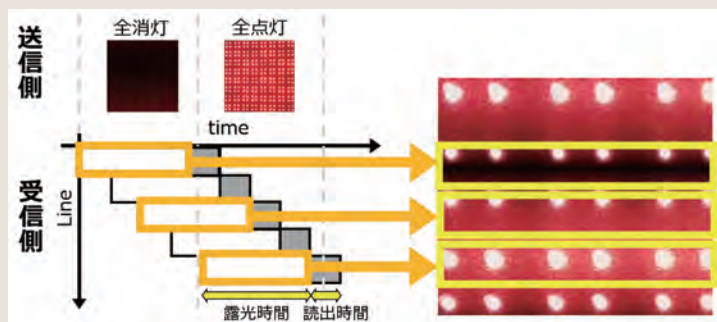
ローリングシャッター方式による可視光通信
