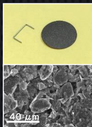
黒鉛負極
