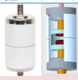
真空インタラプタ
