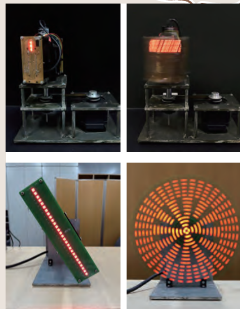
回転式LED送信機
