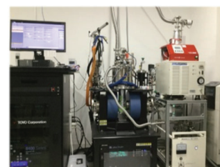
温度可変磁場変調ホール効果測定装置
