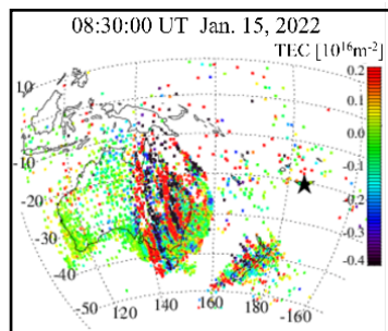
GPS を使った電離圏観測
