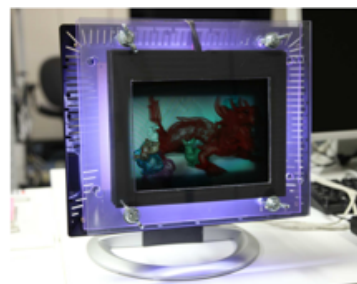
光線再生型 3次元ディスプレイ
