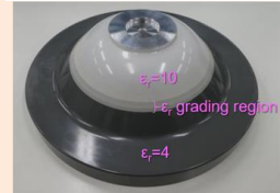
ガス絶縁開閉装置(GIS) 245kV-GIS用FGMスペーサ
