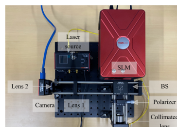
ホログラフィの光学系
