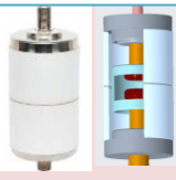
真空インタラプタ
