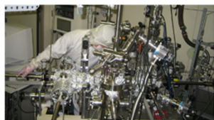
原子層制御CVDシステム
