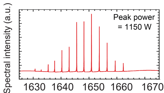
安定化した光周波数コムのスペクトル
